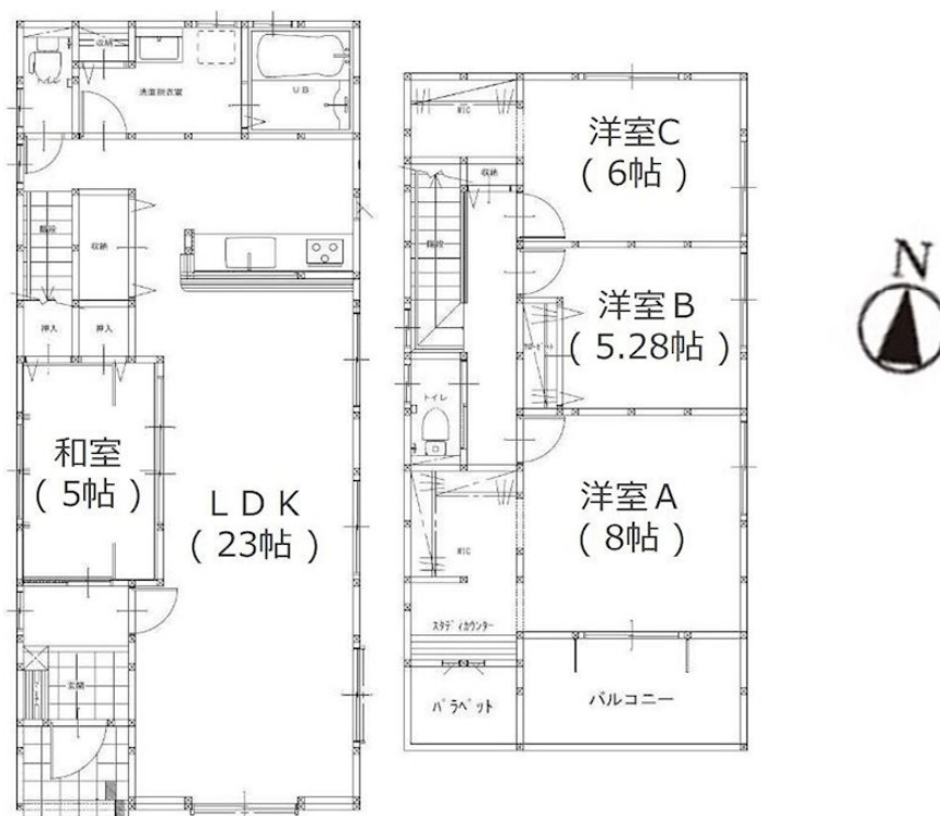
【間取り図】
