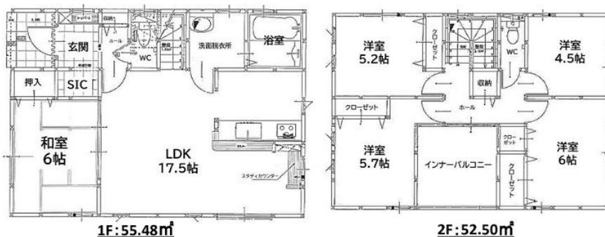
【間取り図】
